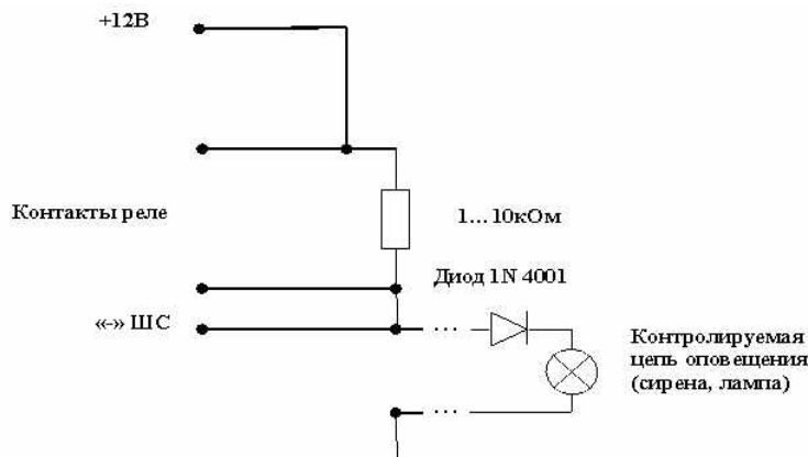
Рис. 25. Схема подключения шлейфа КЦО.
