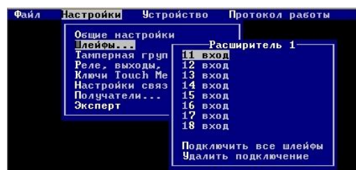
Рис.18. Подключение ШС к входам расширителя на 1 входе ППКОП
