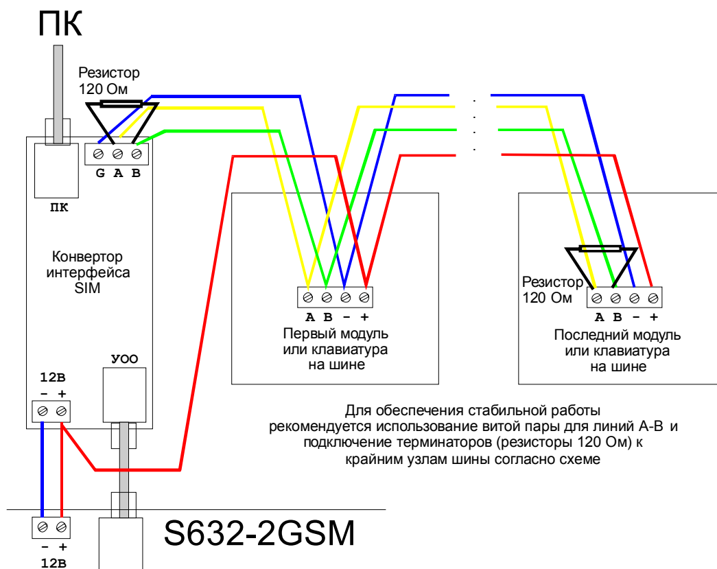
Рис. 57. Подключение устройств по шине RS-485.
