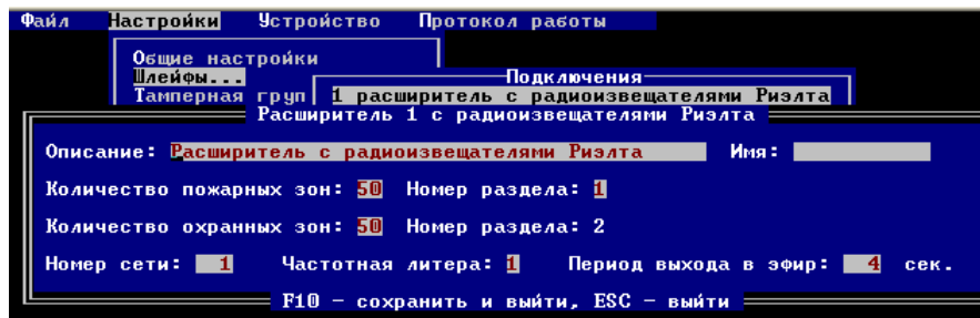
Рис. 28. Настройка расширителя радиодатчиков Ладога-РК.
